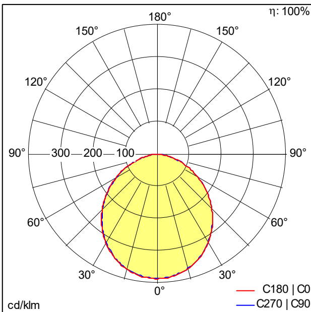
TE_AMY_VARIO_FLEX_220_1950_840_FLEX1.ltd
