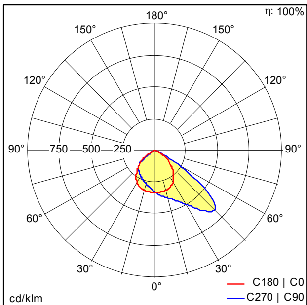
TE_LEO_LED_FL_IP66_210W_840_PC.ltd
