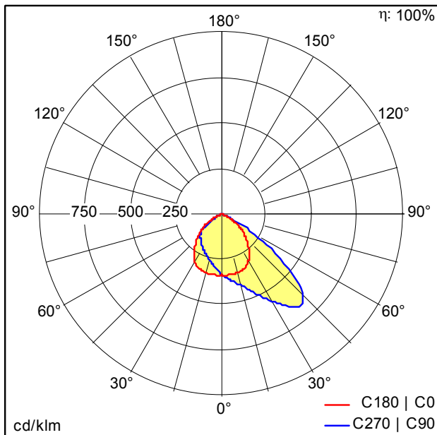
TE_LEO_LED_FL_IP66_200W_840_PC.ltd
