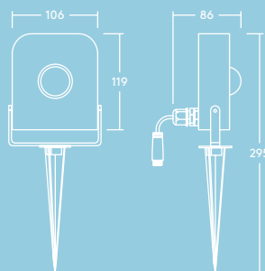
Senzor PIR/Celulă fotoelectrică
